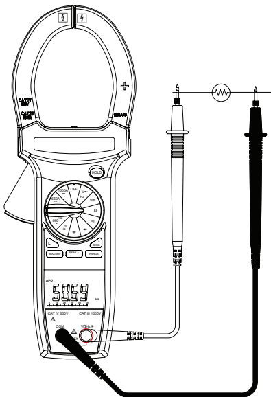
Fig 5. Motstånd \ Kontinuitet \ Diod
