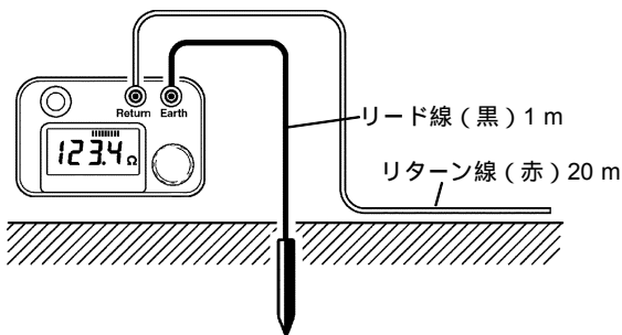
図3 接続図
